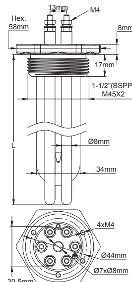
Con accesorio 1½" RPA o rosca M45 x 2
